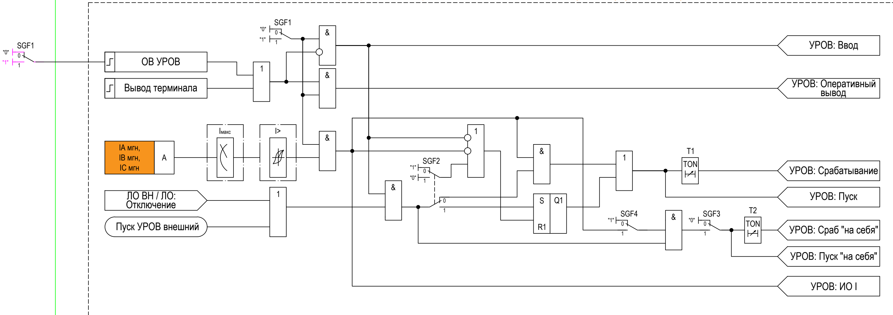
Устройство резервирования при отказе выключателя (УРОВ) (TPRBRF) RBRF1
